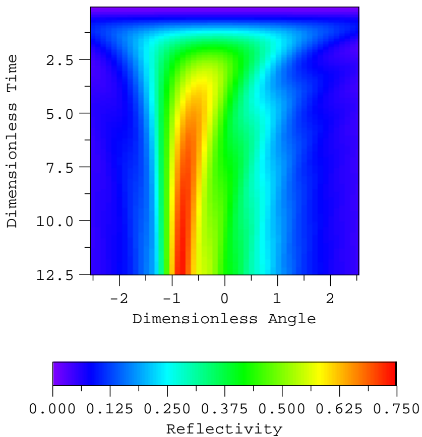
(d) g=-0.5, k=0.49
